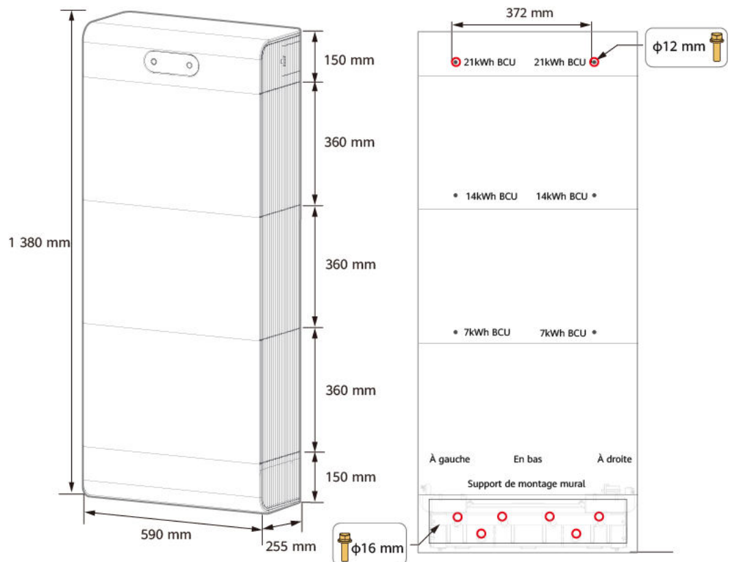
Figure 4-5 Dimensions pour le montage mural
