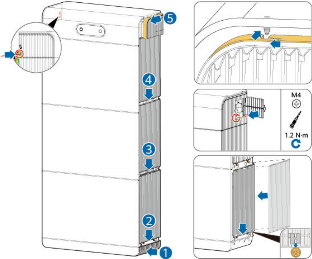
Figure 5-7 Installation des caches décoratifs
