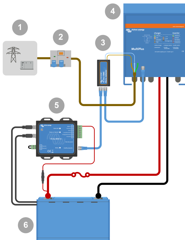
Exemple de câblage de détecteur CA.
