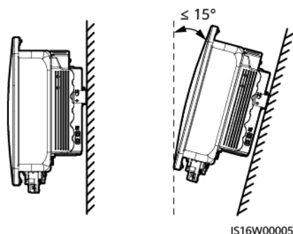
Figure 4-1 Angle d'installation
