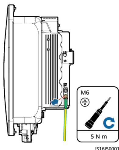
Figure 5-3 Connexion d'un câble PE
