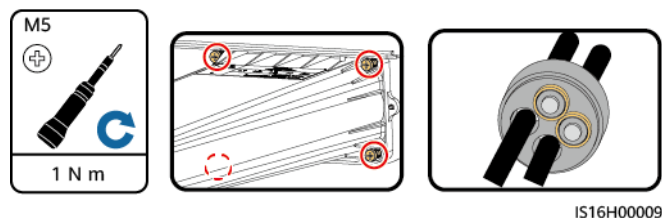
Figure 5-11 Installation d'un boîtier de raccordement
