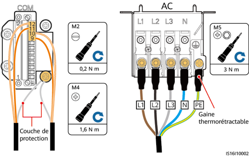
Figure 5-9 Installation des câbles d'alimentation de sortie CA et des câbles de signal
