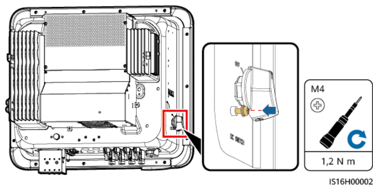
Figure 4-8 Installation de la vis de verrouillage du commutateur CC
