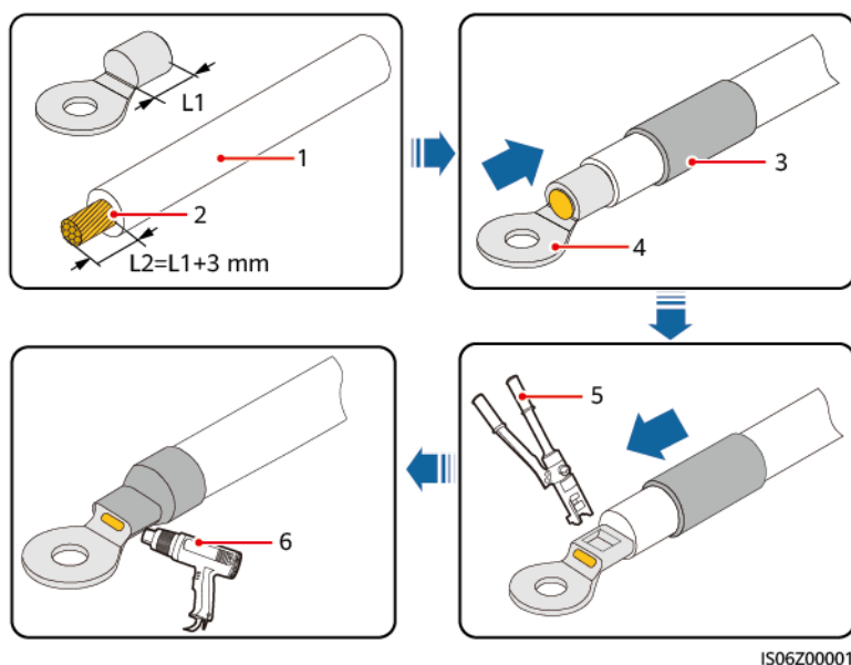
Figure 5-2 Sertissage d'une cosse OT
