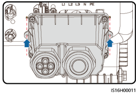
Figure 4-9 Alignement des broches de positionnement
