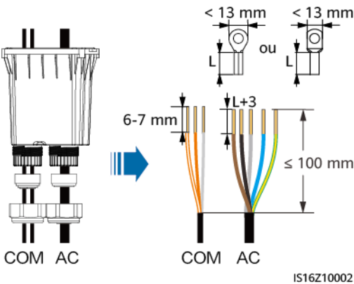
Figure 5-8 Acheminement des câbles
