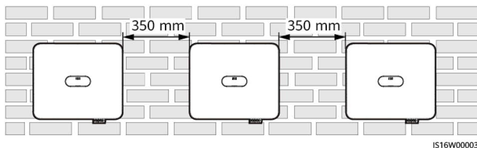
Figure 4-3 Installation horizontale (recommandée)
