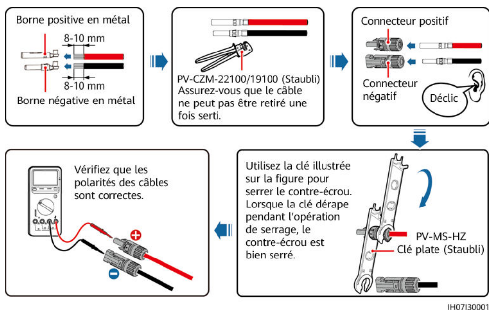
Figure 5-5 Assemblage des connecteurs CC
