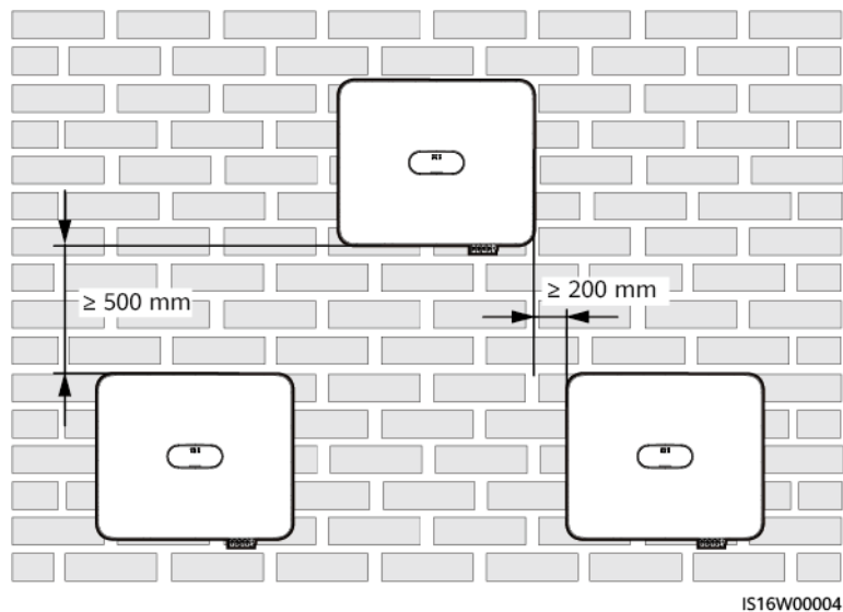
Figure 4-4 Installation en triangle (recommandée)
