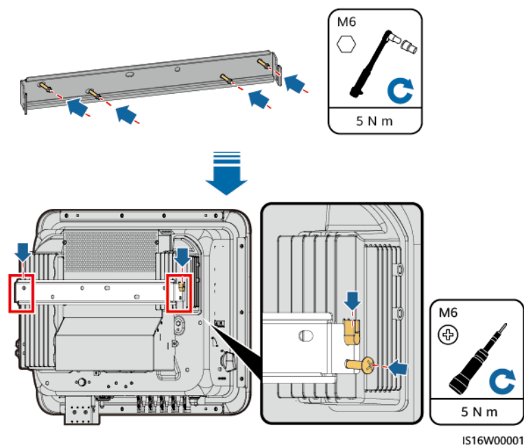
Figure 4-7 Installation d'un onduleur
