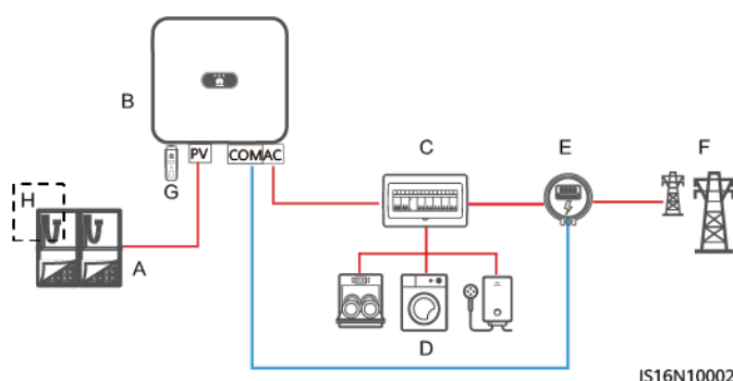
Figure 2-3 Application de mise en réseau (onduleur simple)
