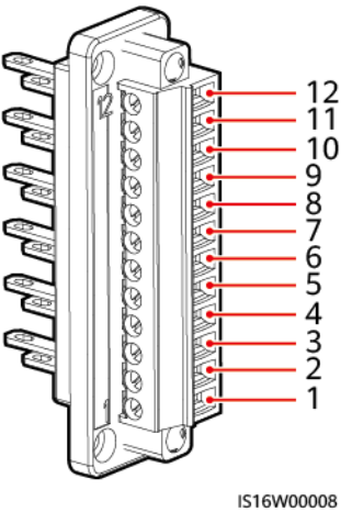
Figure 5-7 Définitions des signaux
