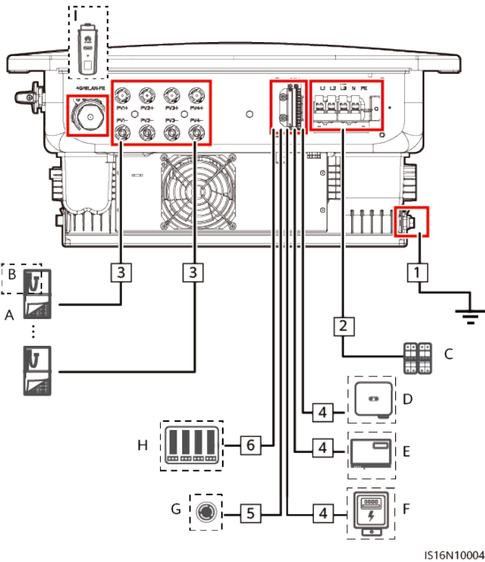
Figure 5-1 Connexions de câbles SUN2000 (Les composants des cases en pointillés sont optionnels.)
