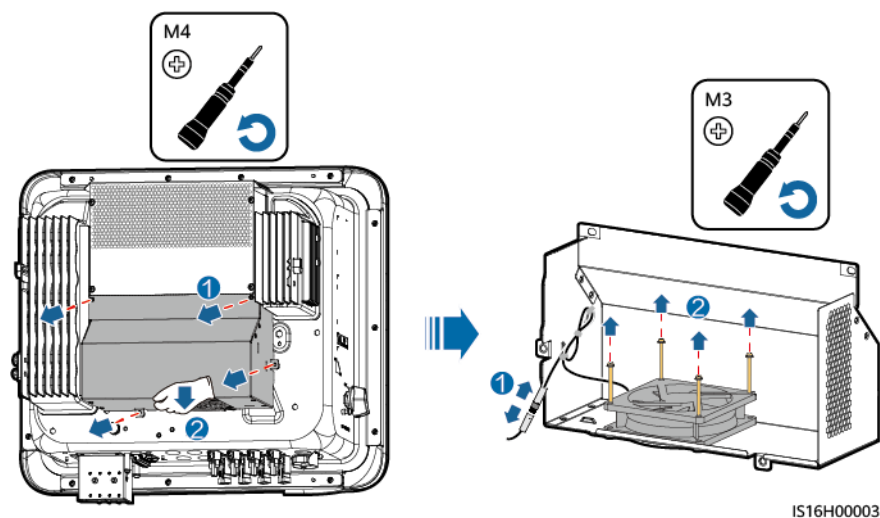
Figure 8-1 Retrait d'un ventilateur défectueux
