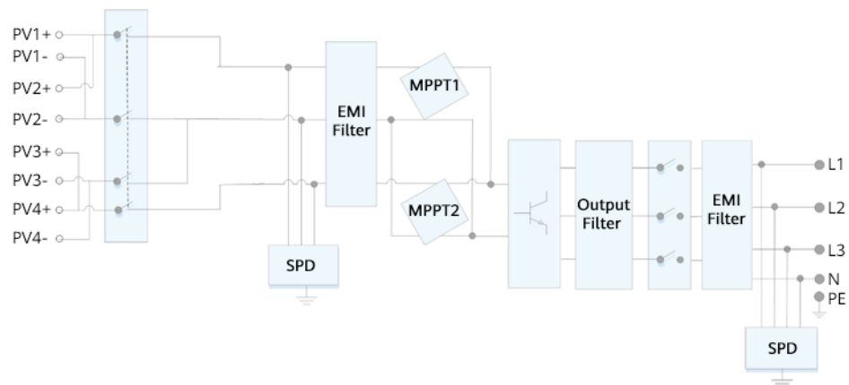
Figure 2-6 Schéma conceptuel
