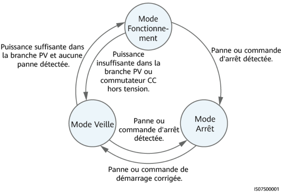
Figure 2-5 Modes de fonctionnement
