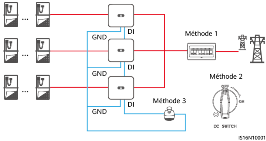
Figure E-2 Méthodes de déclenchement d'un arrêt rapide
