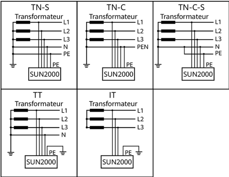
Figure 2-2 Réseaux électriques pris en charge
