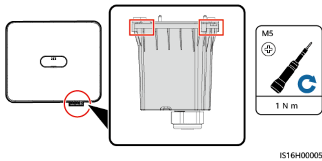
Figure 4-10 Installation d'un boîtier de raccordement
