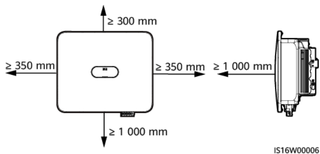
Figure 4-2 Dégagement
