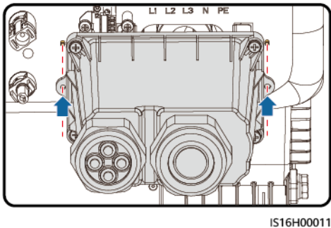
Figure 5-10 Aligement des broches de positionnement
